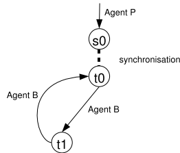
Fig. 11. Encoding iterate
