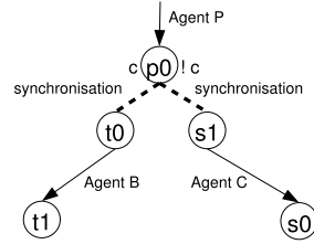
Fig. 10. Encoding if-then-else
